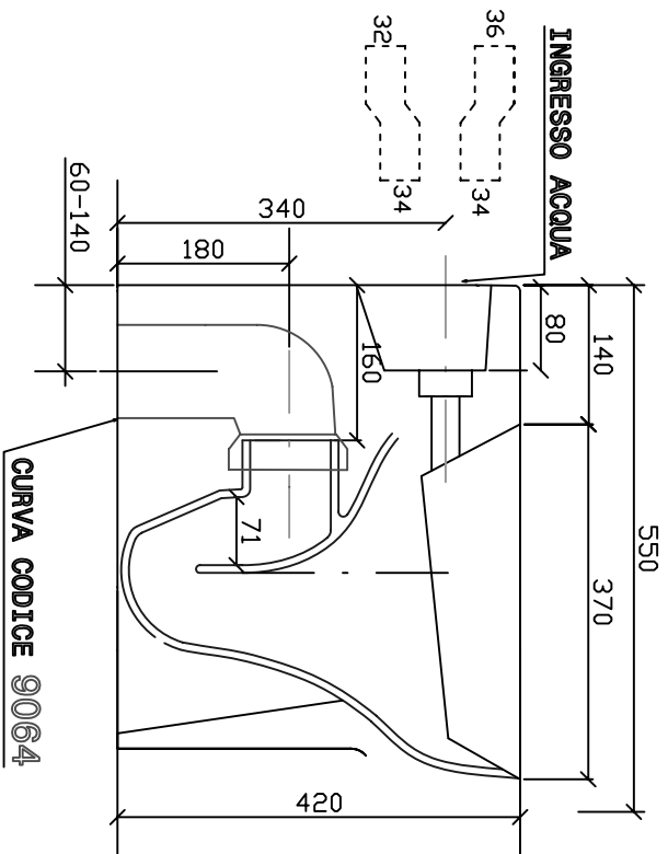
SCARICO PAVIMENTO 60mm-140mm
